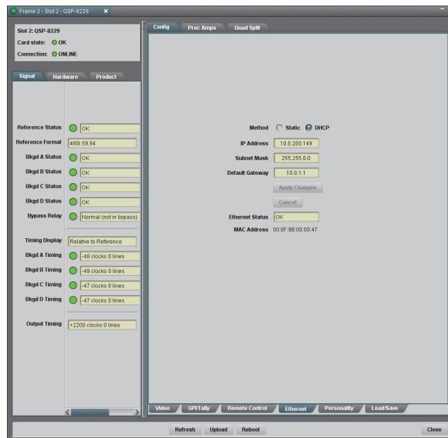
Config Tab — Ethernet Tab
