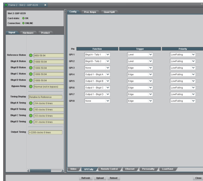
Config Tab — GPI/Tally Tab
