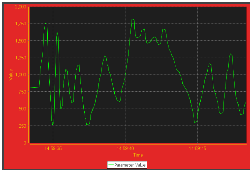
Figure 3.43 - WIDGET_GRAPH Hint
