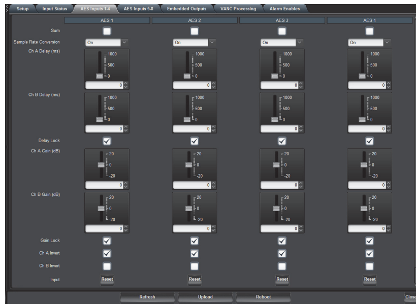
AES Inputs 1-4 Tab
