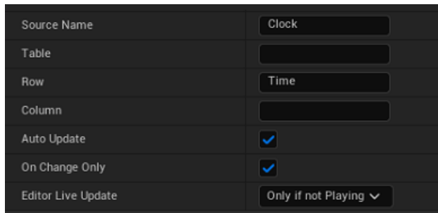
DataLinq - Summary
