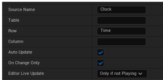
DataLinq - Summary
